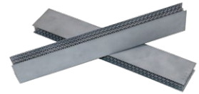
卫星轻量化结构组件 铝合金 320mm*58mm*20mm
